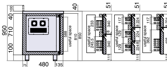
A-A
